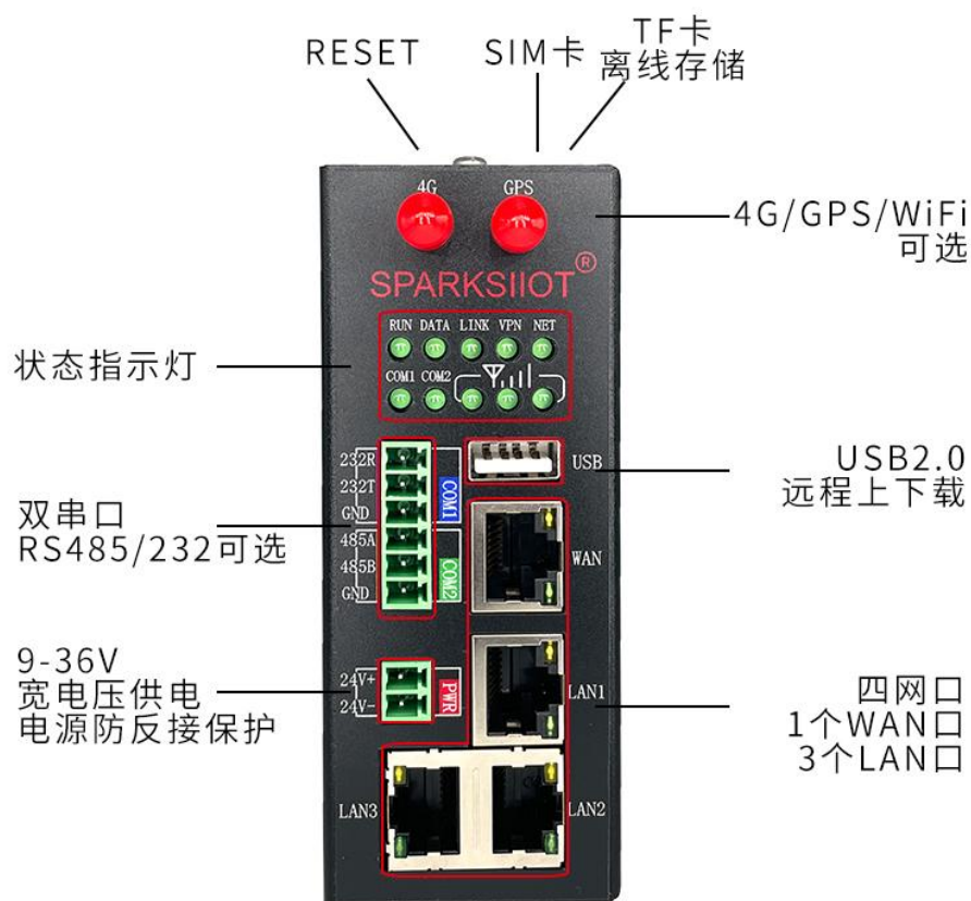
图：星原物联网网关 G 系列接口说明
